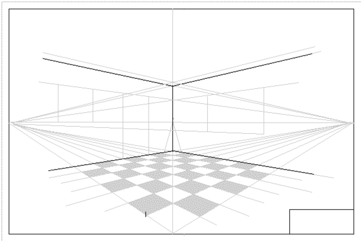
ใช้เส้นจริงเขียนเพื่อให้เห็นภาพรวมชัดเจน และวางตำแหน่งของหน้าต่าง
